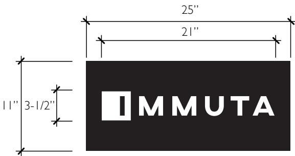
SIGN DETAIL SCALE: 1/2" = 1'-0"
