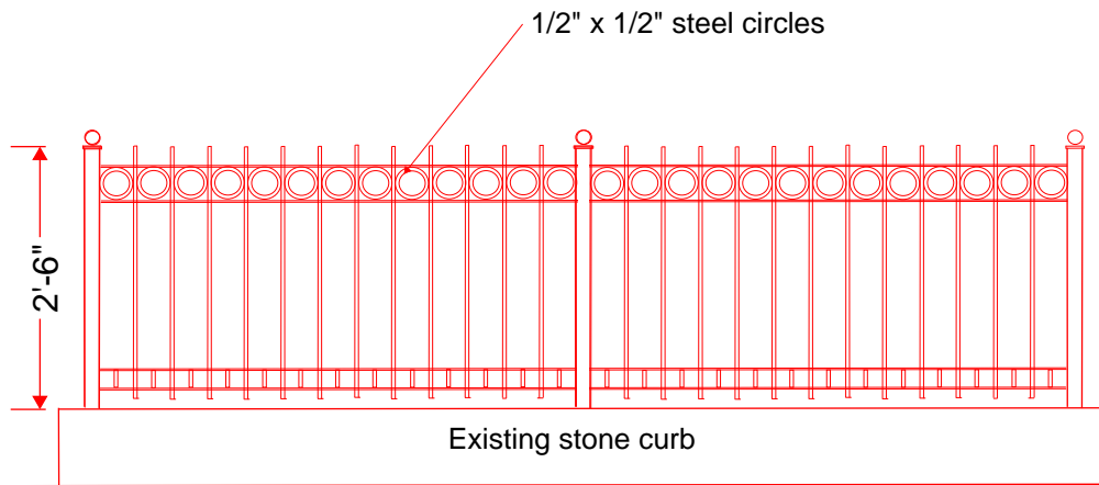
ELEVATION
