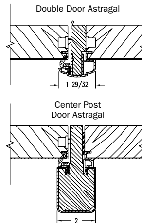
Astragal
