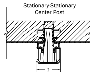
Astragal
